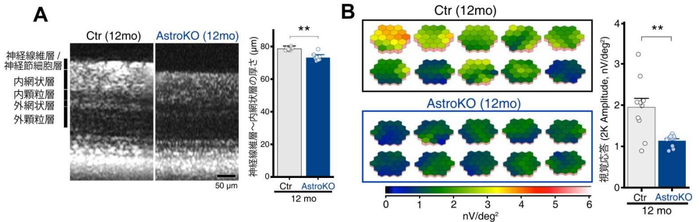
図 6. AstroKO マウスは緑内障様症状を示す
